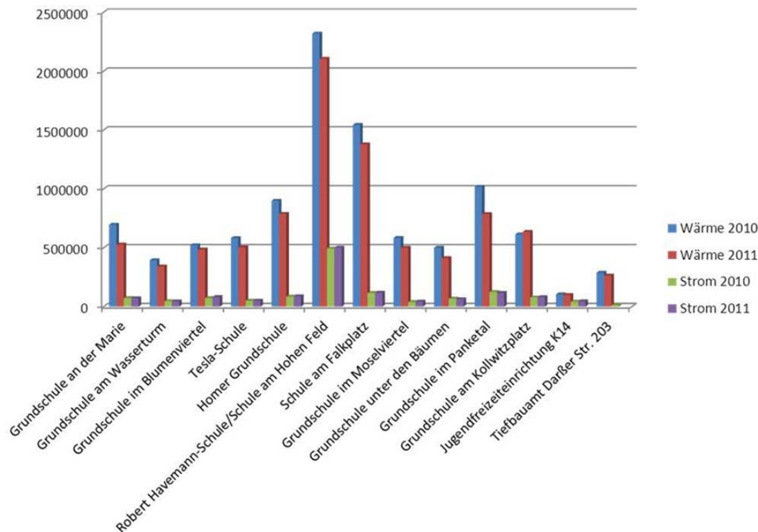
Wärme- und Stromverbrauch im Vergleich 2010 und 2011 unbereinigt (in kWh)
